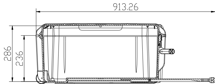
截面 X-X
